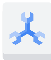
Spanner
